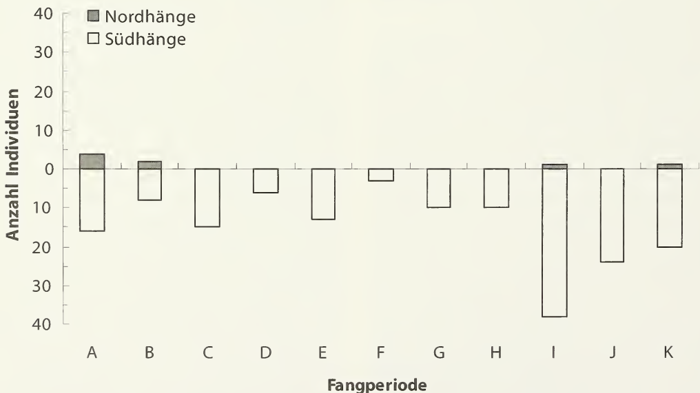
Abb. 10: Anzahl Lycosidae (inkl. juvenile Tiere) an den Nord- und Südhängen in den Fangperioden A-K (12.09.2007 - 27.04.2008); genaue Daten zu den Fangperioden vergl. Anhang 2.
